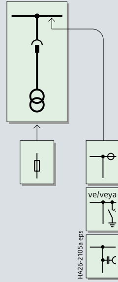
Ölçü panosu
