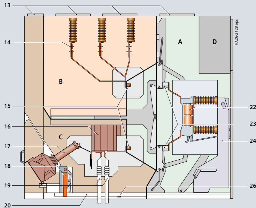
Serbest-dikili, genişlik: 1200 mm, derinlik: 2700 mm, kablo bölgesinde primer sigortalı devrilebilir tip GT
