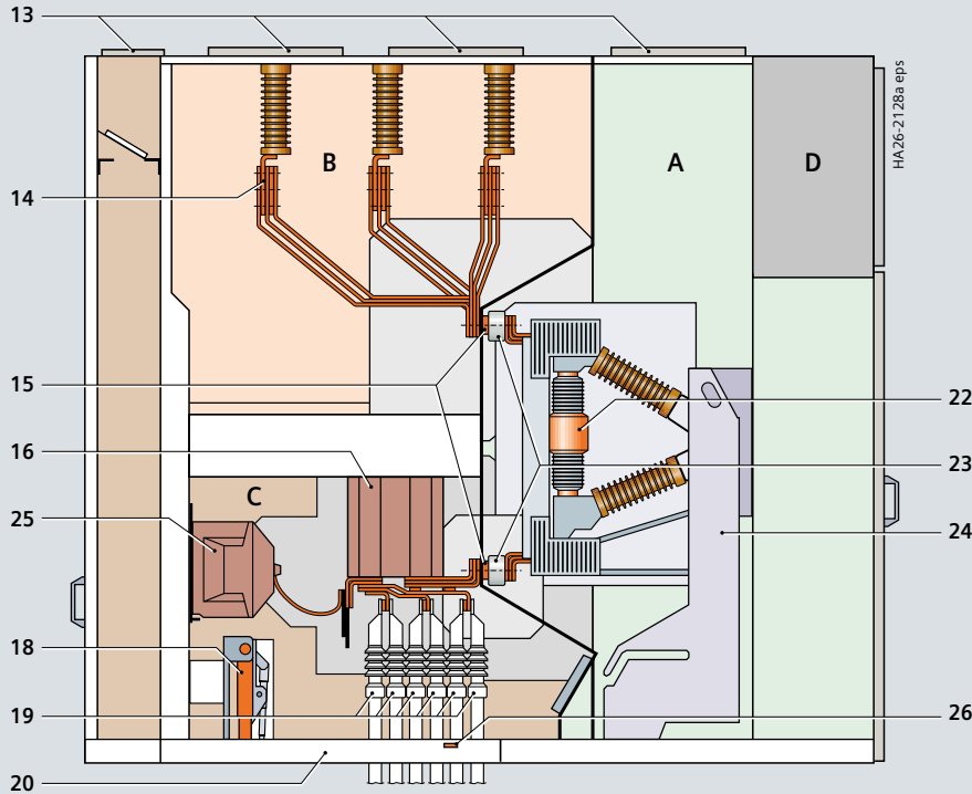
Serbest-dikili, genişlik: 1200 mm, derinlik: 2700 mm, kablo bölgesinde sabit tip GT
