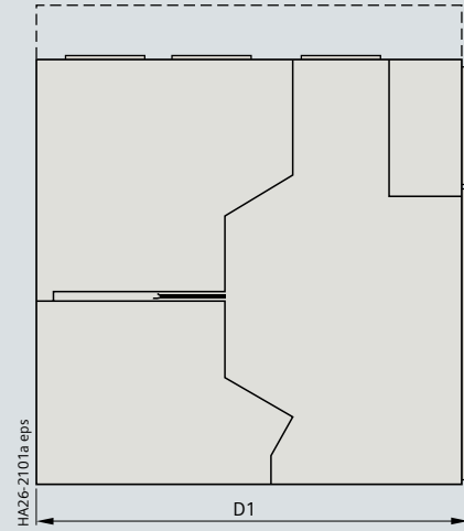
Yandan görünüm (Duvara dayalı)
