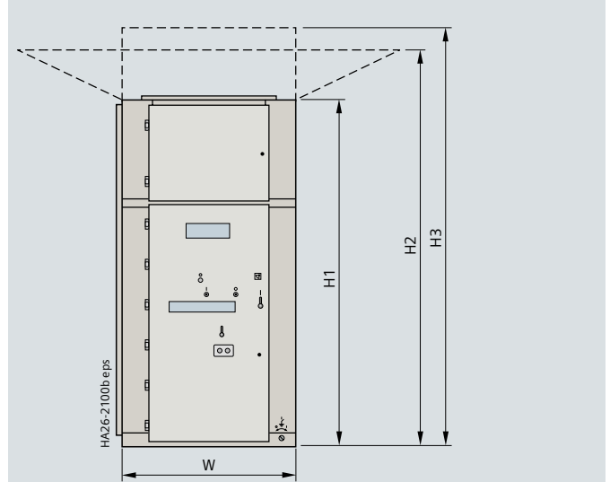
Önden görünüm
