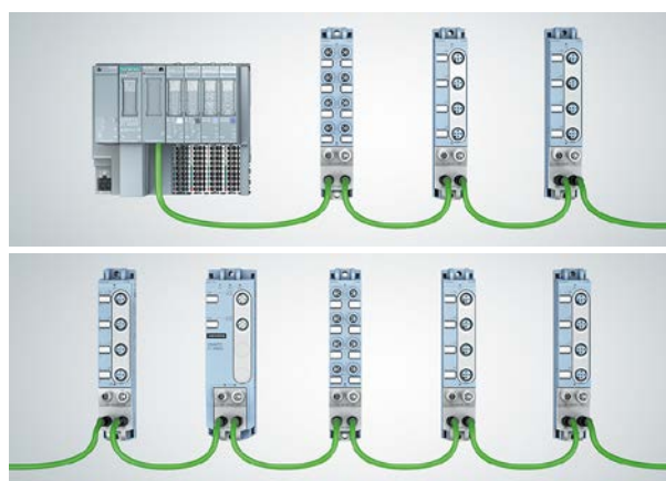
図. ET 200AL 構成方法
